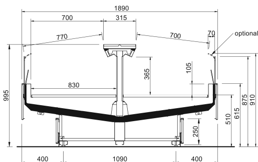
Sezione Silk N_MAX_lineare
