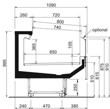
Sezione Silk N_MAX_MT
