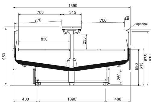
Sezione Silk N_STD_lineare
