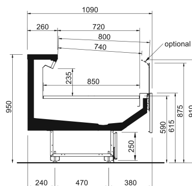
Sezione Silk N_STD_MT
