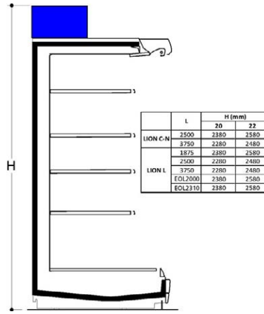
EPTABLU - OPTION
