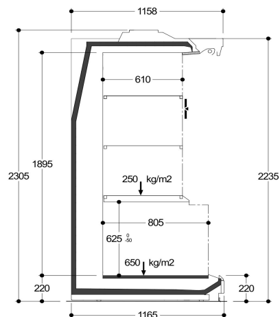
Sezione HD8 22 L copia
