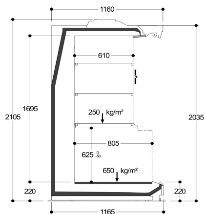
Sezione HD8 20 L copia
