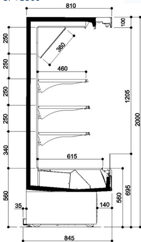
3P+S360
