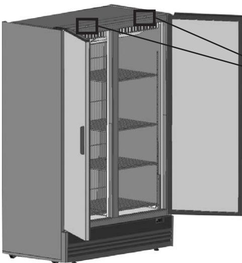
Microinterruptor del ventilador interno (con puerta abierta: ventilador interno non conectado)
