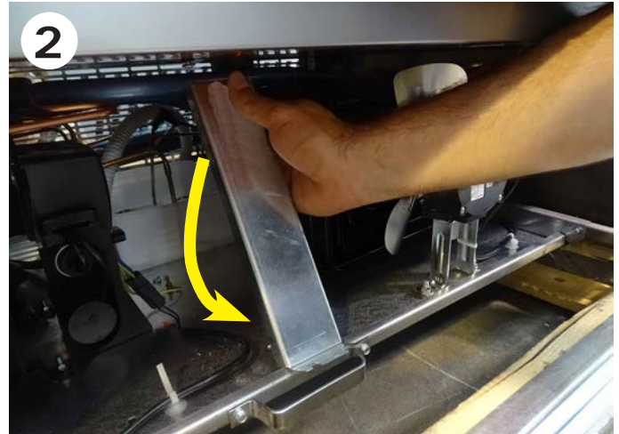
2 RIMUOVERE LA STAFFA SUPPORTO BASAMENTO
