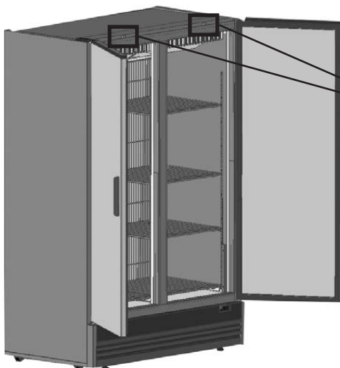
Microinterrupteur du ventilateur intérieur (avec la porte ouverte: ventilateur deconnectée)
