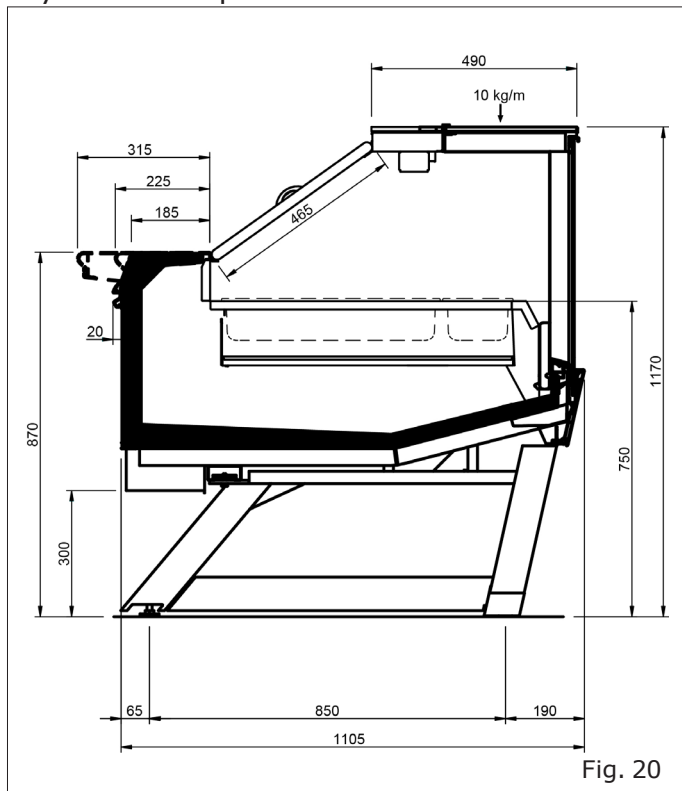
Style RDB con pies
