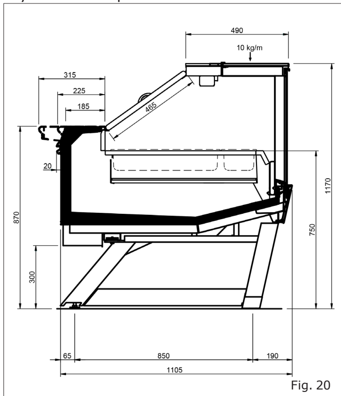
Style RDB avec pieds
