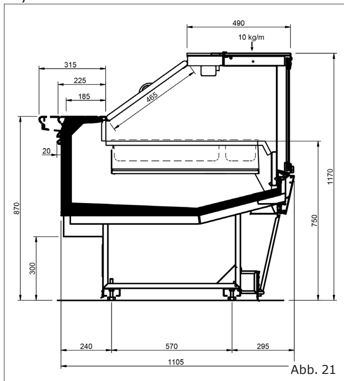
Style WO mit Füßen
