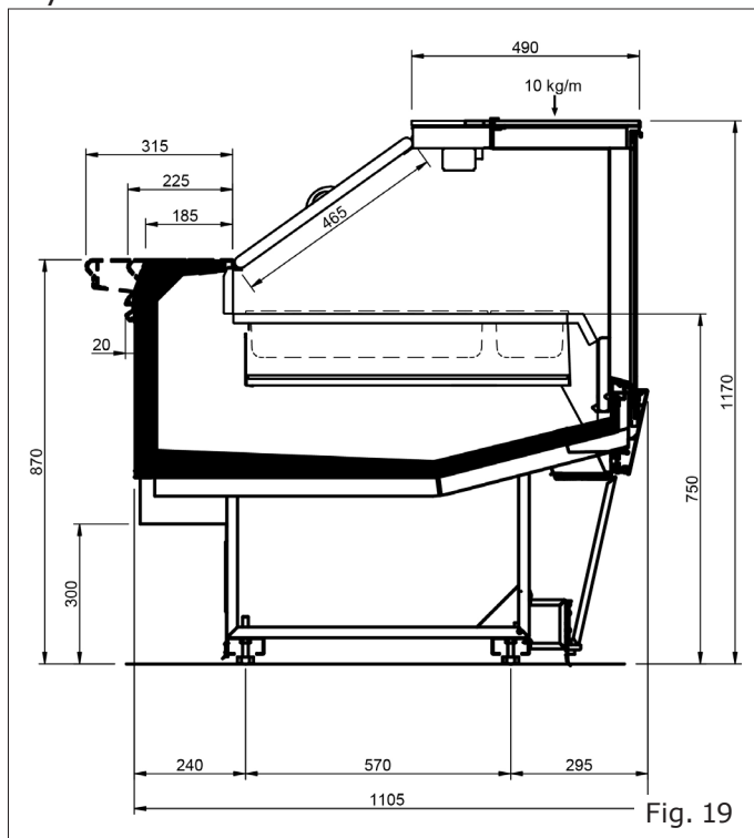
Style RDB com pés
