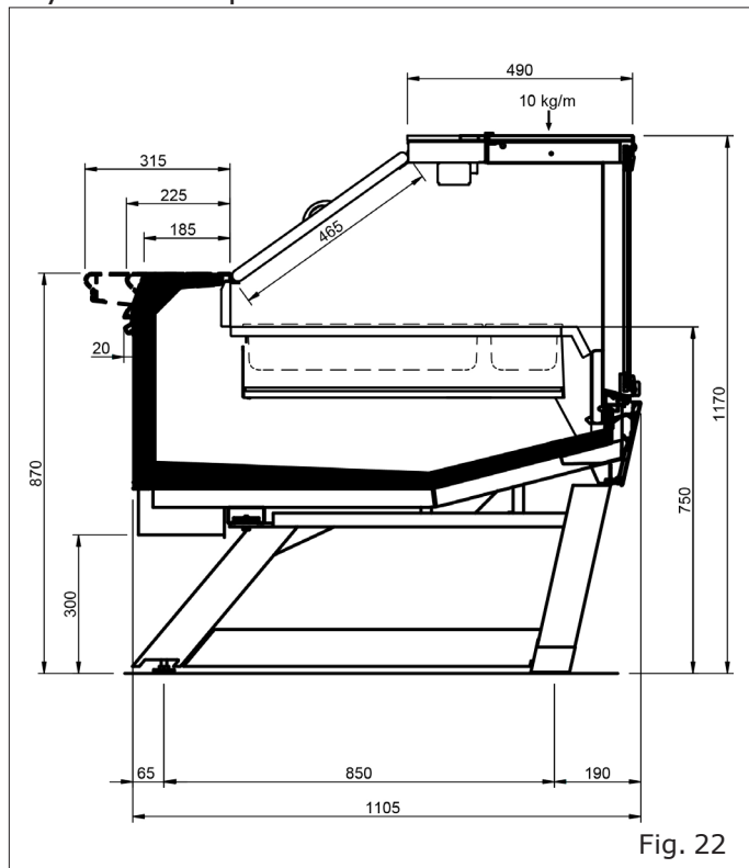
Style WO con piedi
