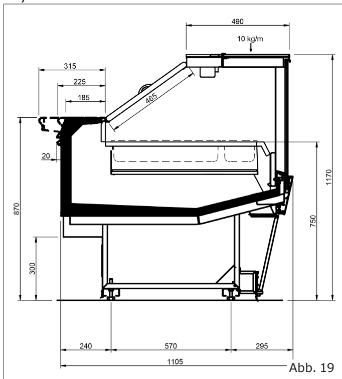
Style RDB mit Füßen
