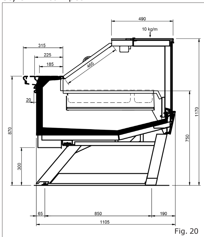
Style RDB com pés
