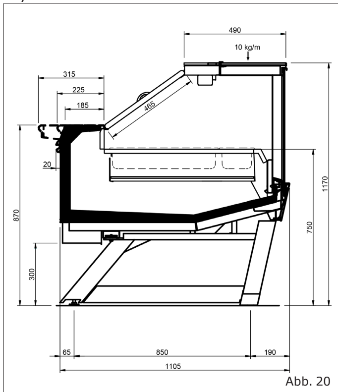
Style RDB mit Füßen
