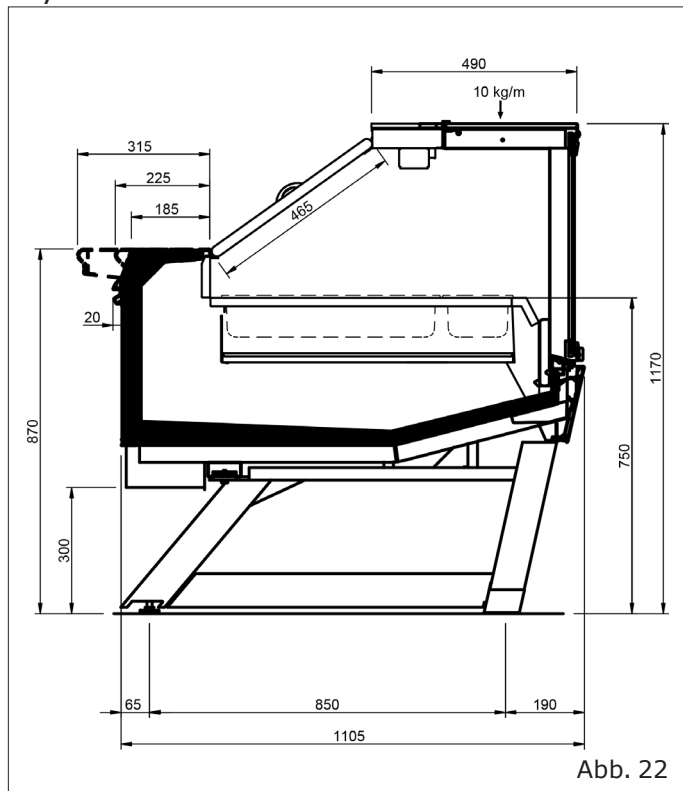
Style WO mit Füßen
