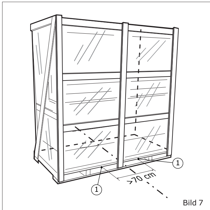
1. Lyftpunkter
