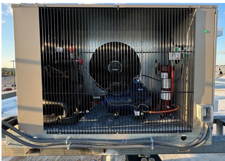
Figure 2.2 ECO 2 Mini Condensing Unit
