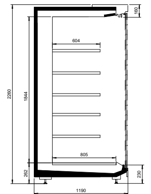
NordicLine MD7 25-119-226 GD
