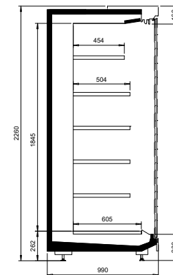
NordicLine MD7 25-99-226 GD
