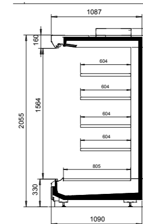
NordicLine MD5 30-109-206
