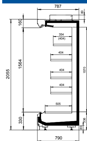
NordicLine MD5 30-79-206
