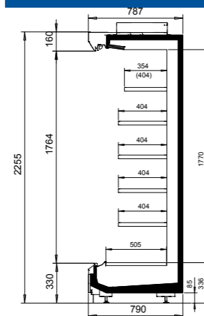
NordicLine MD5 30-79-226
