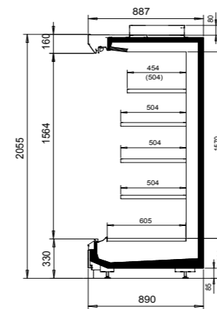
NordicLine MD5 30-89-206
