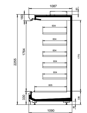
NordicLine MD5 30-109-226
