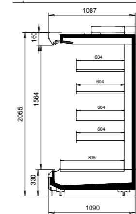
NordiLine MD5 30-109-206
