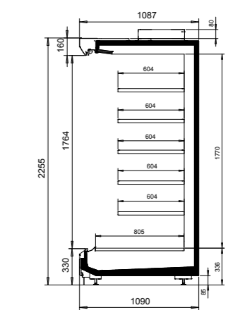
NordiLine MD5 30-109-226
