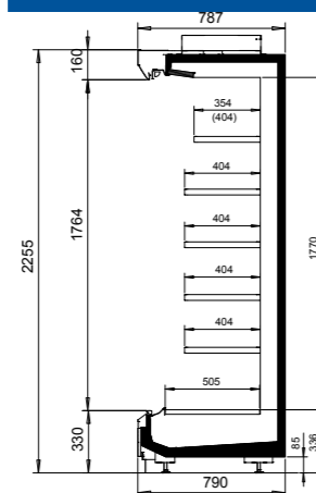
NordiLine MD5 30-79-226
