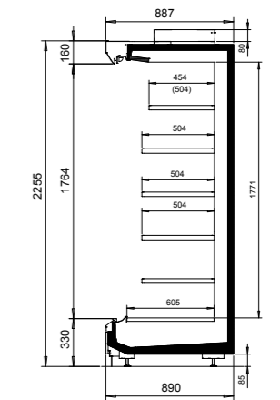
NordiLine MD5 30-89-226
