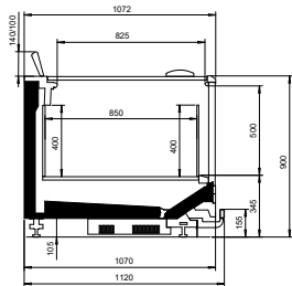
NordicLine IS7 100-90 flat lids
