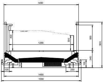
NordicLine IS7 150-90 SB CO open
